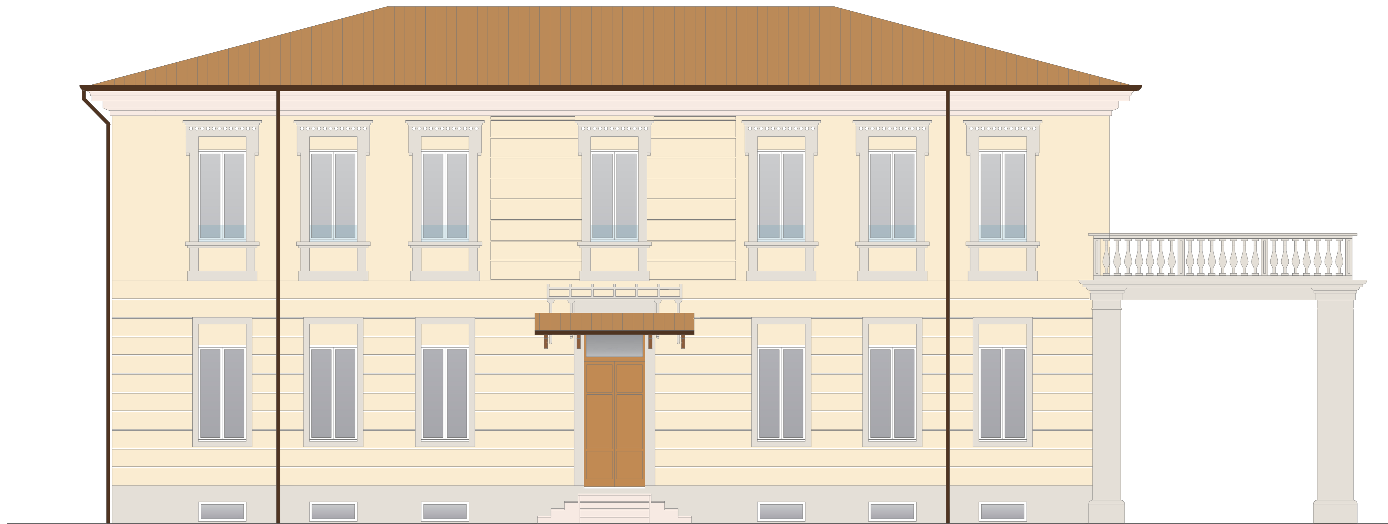
PROSPETTO FRONTE EST stato di fatto - scala 1:50
