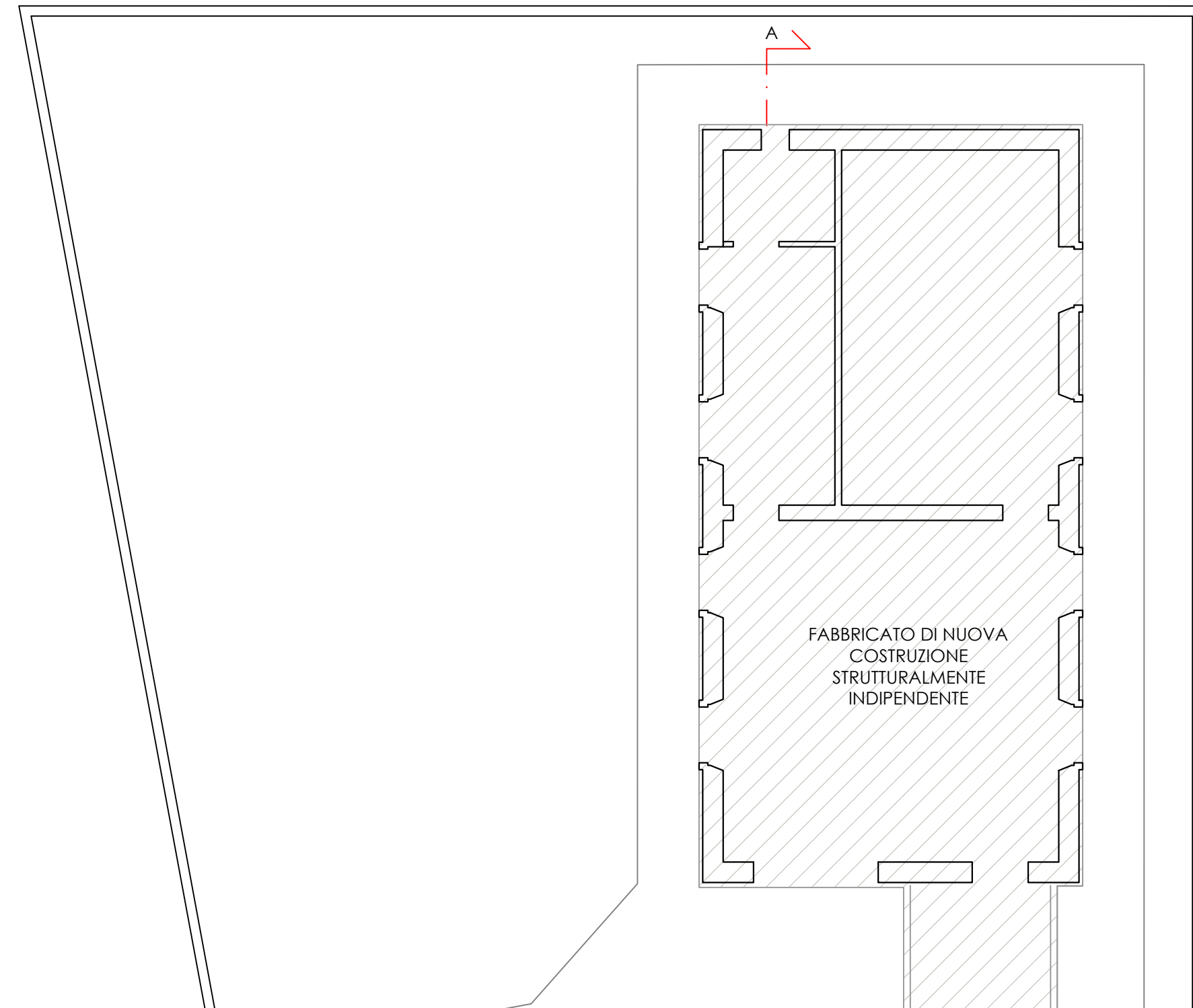
PIANTA PIANO RIALZATO progetto - scala 1:100
