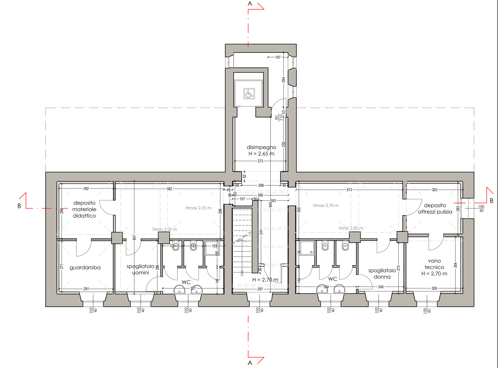
PIANTA PIANO INTERRATO progetto - scala 1:100
